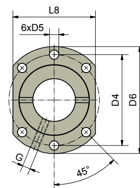
Hole pattern 1 to DIN 69051
