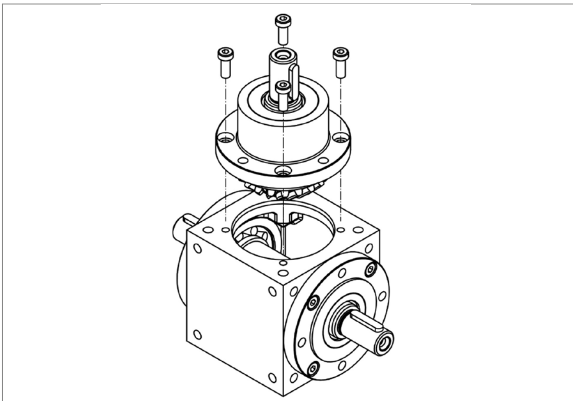
Abb. 8: Ein-/Ausbau Lagerflansch
