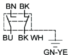
Afb. 15: Elektrisch aansluitschema voor eindschakelaar
