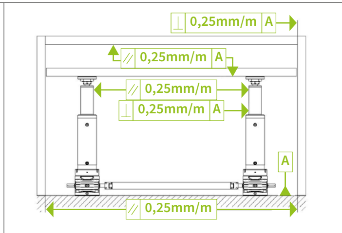
Fig. 6: Installatienauwkeurigheid: evenwijdigheid en loodrechtheid
