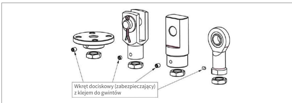
Rys. 9: Po ustawieniu położenia należy przykręcić i zabezpieczyć części takie jak kołnierz mocujący, głowica widelkowa, głowica wahliwa.
