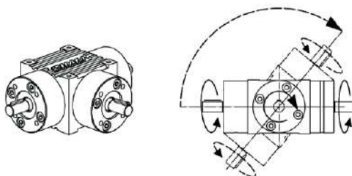
Rys. 11: Wersja T (przekładnia kątowa)
